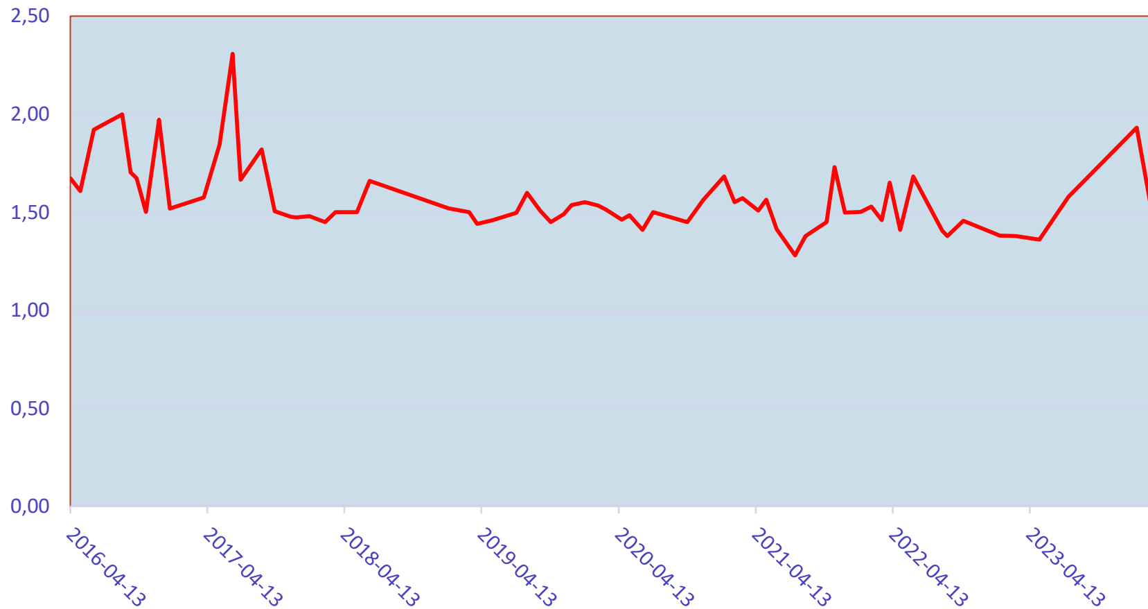
Stężenie ^{85}\text{Kr} w próbkach pobranych w Warszawie w latach 2015-2023 [Bq/m 3 ]
