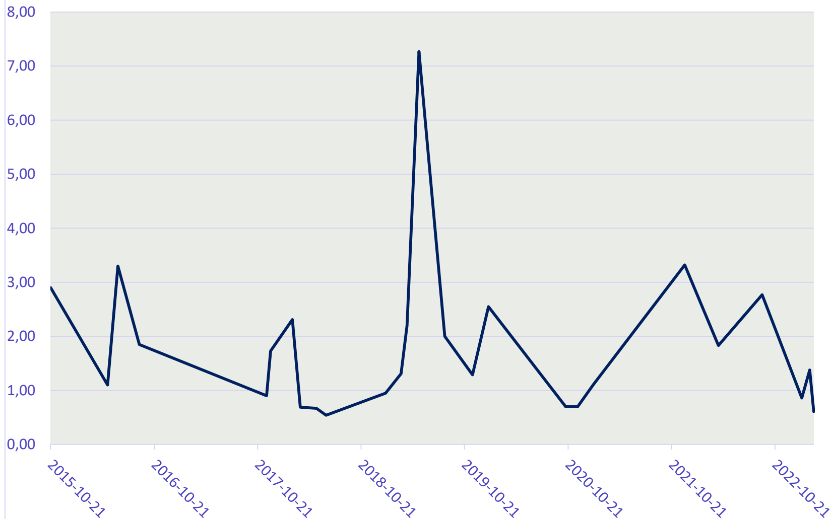
Stężenie ^{133}\text{Xe} w próbkach pobranych w Warszawie w latach 2015-2023 [mBq/m 3 ]
