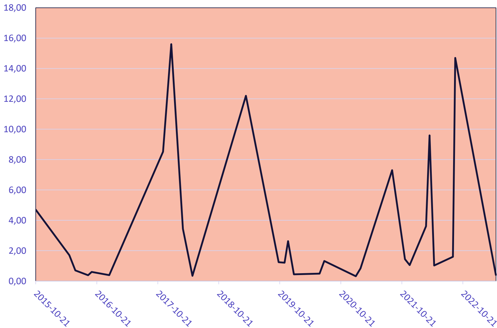
Stężenie ^{131m}\text{Xe} w próbkach pobranych w Warszawie w latach 2015-2023 [mBq/m 3 ]
